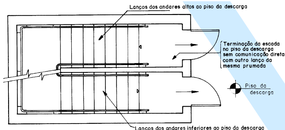
Figura 3 - Segmentação das escadas no piso da descarga
