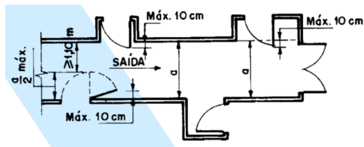
Abertura de portas no sentido do trnsito de sada: Imagem exemplificativa
