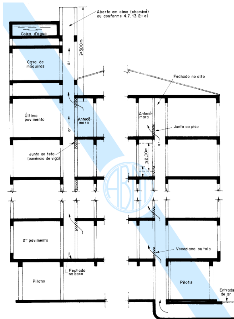
Imagem da NBR 9077 exemplificando os dutos de entrada e sada de ar em uma vista de corte.
