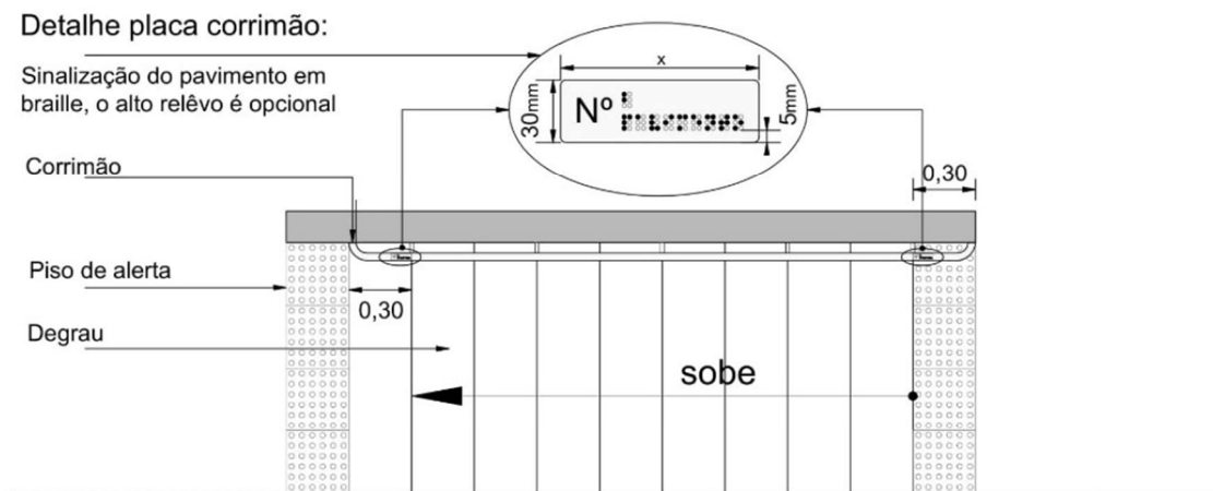
Figura 63 – Sinalização de corrimão – Vista superior
