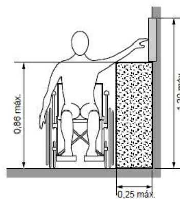
Figura 14 – Alcance manual lateral sem deslocamento do tronco
