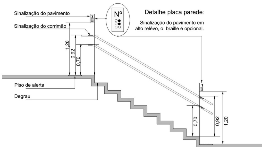
Figura 64 – Sinalização de pavimento – Vista lateral
