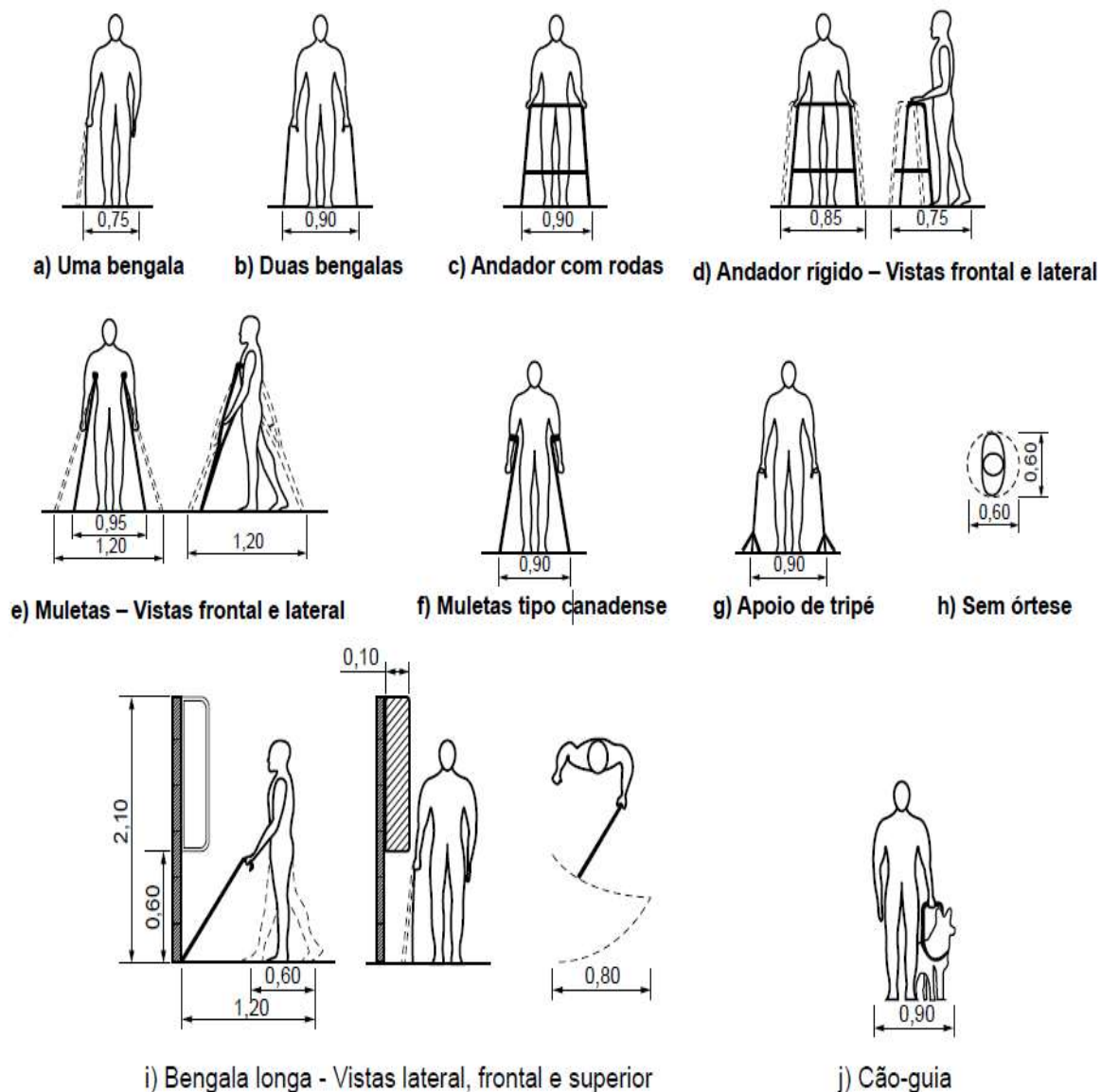
Figura 1 – Dimensões referências para descolamento de pessoa em pé
