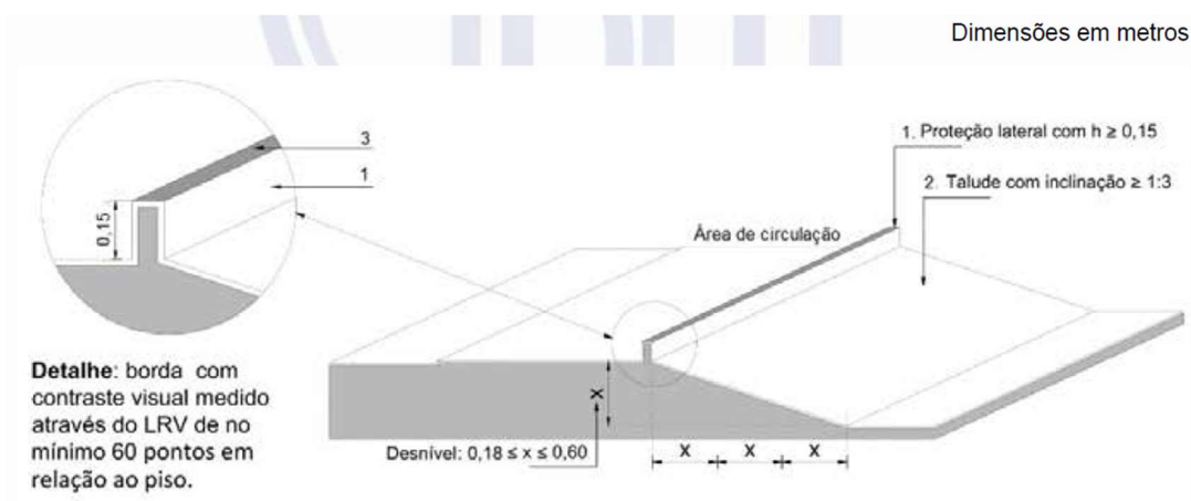
Figura 10 – Proteção contra queda em áreas de circulação com implantação de margem plana
