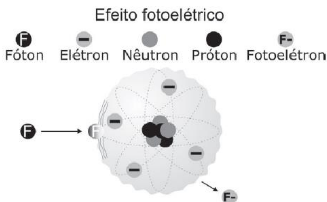
Efeito fotoelétrico. Imagem retirada de: WATANABE, Plauto Christopher Aranha; ARITA, Emiko Saito. IMAGINOLOGIA E RADIOLOGIA ODONTOLÓGICA. 2. ed. Rio de Janeiro: Elsevier, 2019. 568 p.
