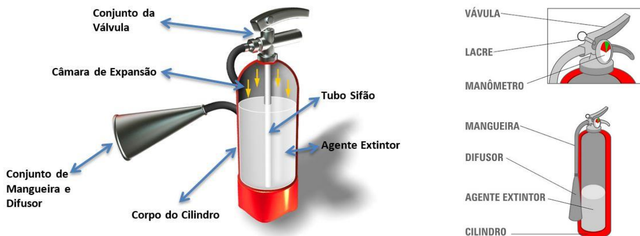
Figura 1.4: principais itens auxiliares dos dispositivos extintores.
